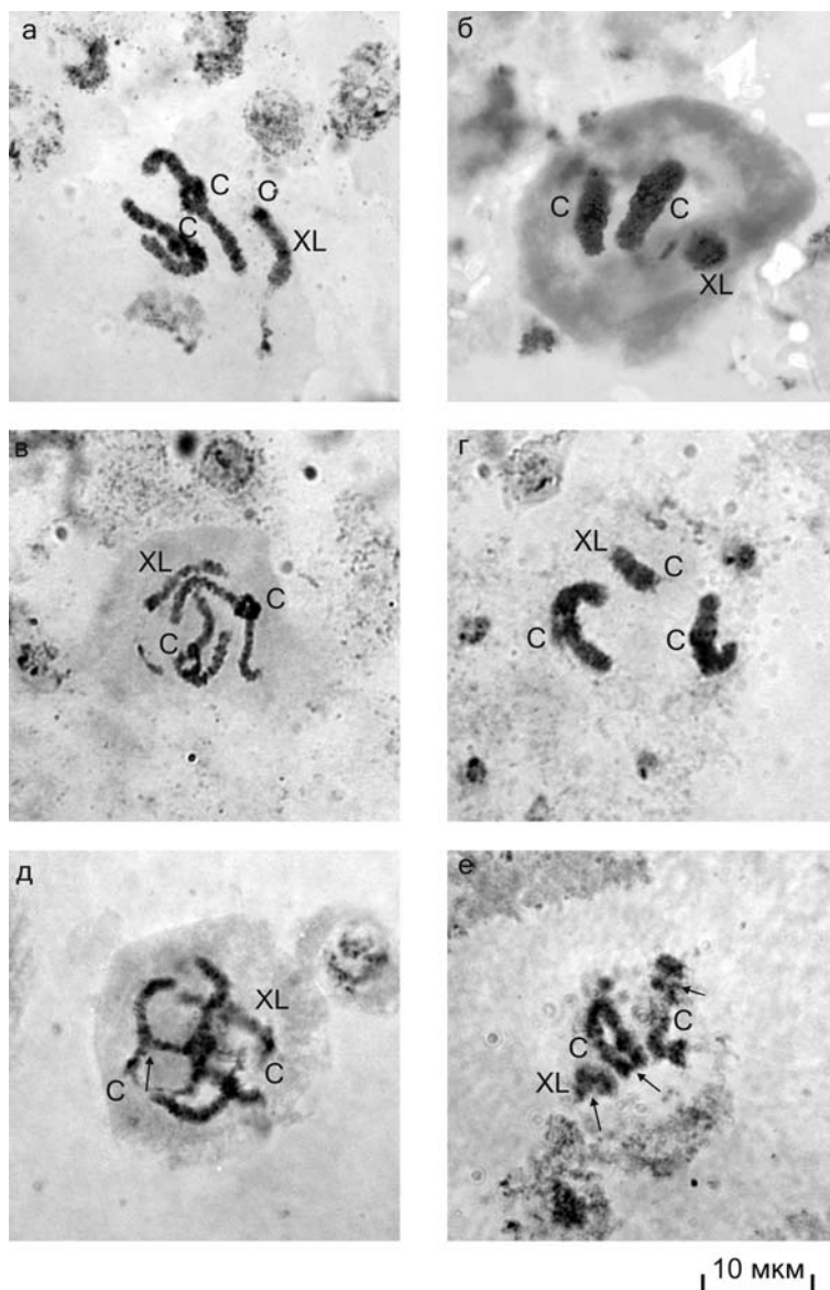
Рисунок 1 – Расположение хромосом в ядре: а, б – Drosophila santomea , в, г – D. yakuba , д, е – гибрид D. yakuba x D. santomea . XL – левое плечо X-хромосомы, С – центромерный район, стрелками указаны участки асинapsирования гомологов
