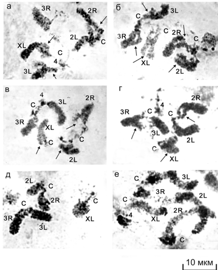
Рисунок 2 – Первичные политенные хромосомы трофоцитов яичников D. melanogaster . Гибриды в P-M системе гибридного дисгенеза: а, б – Canton S x \pi_2 ; в – Berlin x \pi_2 ; г – \pi_2 x Berlin . Линии: д – Canton S ; е – \pi_2 . XL, 2R, 2L, 3R, 3L, 4 – хромосомные плечи, С – центромерный район, стрелками указаны участки асинапирования гомологов
