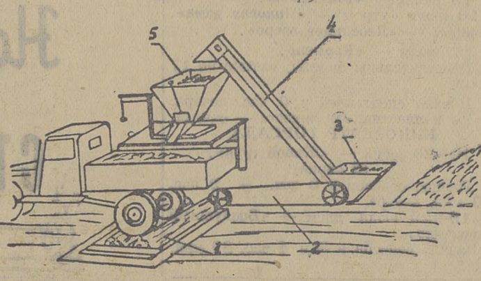
1. Деревянные бревна. 2. Ремённый привод. 3. Приемный ковш. 4. Элеватор. 5. Приемный бункер.
