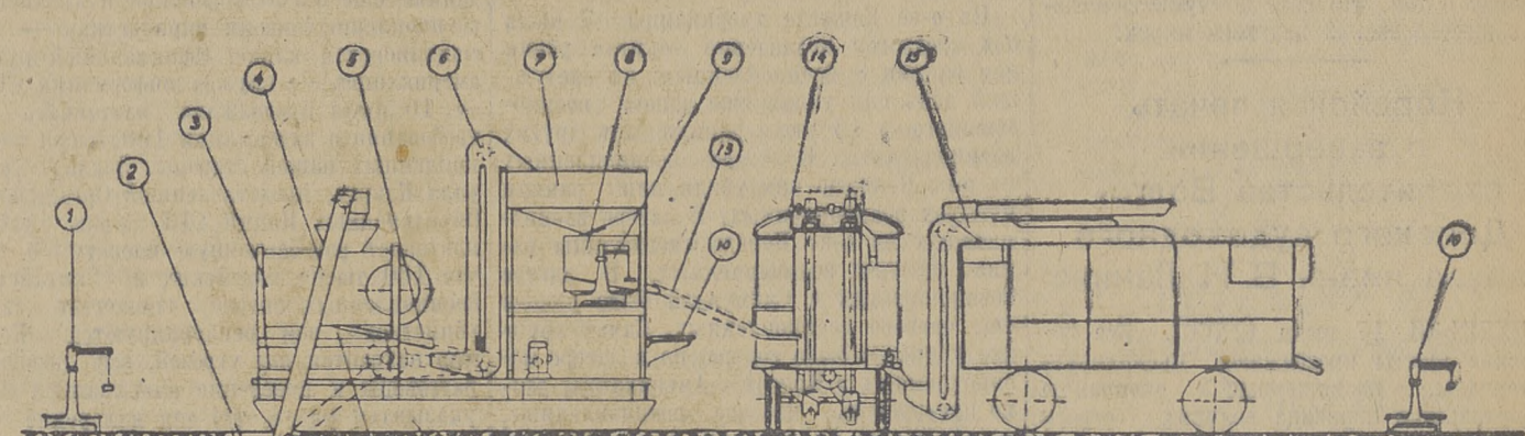
1. Весы приемочные в 1 тонну. 2. Загрузочный ковш. 3. Вейлка-сортировка «BC-2». 4. Загрузочный элеватор. 5. Наклонные щитки. 6. Элеватор чистого зерна. 7. Большой бункер. 8. Малый бункер. 9. Весы грузоподъемностью в 1 тонну. 10. Откидная площадка. 11. Подставка. 12. Сани. 13. Лоток. 14. Зерносушилка «Кузбасс». 15. Зерноочистительная машина «OC-3». 16. Отгрузочные весы.
