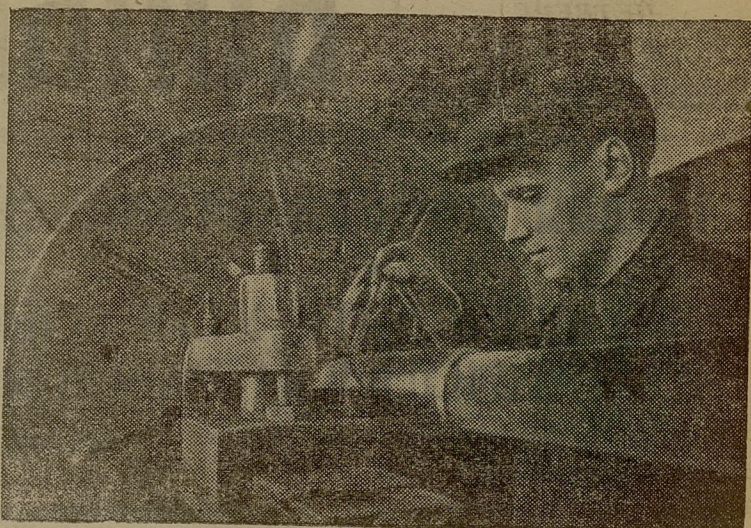
А. С. Реунов — стахановец токарь механического цеха судоремонтного завода им. 25 Октября Верхне-Волжского речного пароходства обрабатывает гребной вал для теплохода «Газовец». А. С. Реунов выполняет до 300 процентов нормы. (Фотохроника ТАСС)
